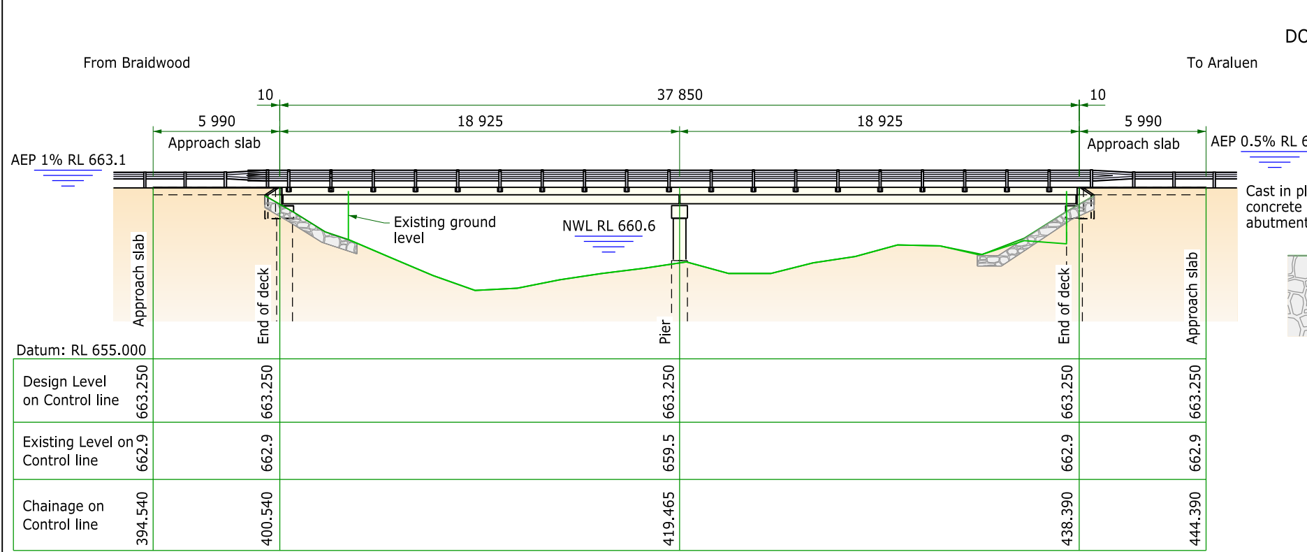
ELEVATION 1:250
