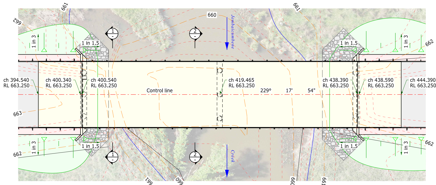
PLAN 1:250
